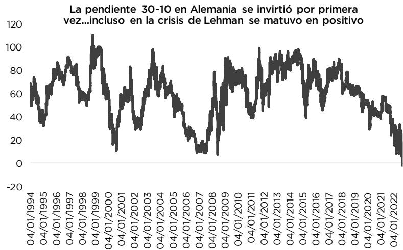
GRÁFICO 1. Inversión de la pendiente 30-10 en Alemania
